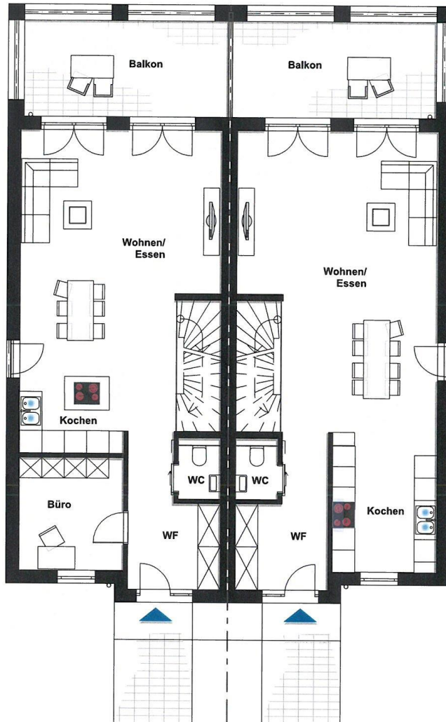
Erdgeschoss mit Keller (ca. 67,00 m 2 )
